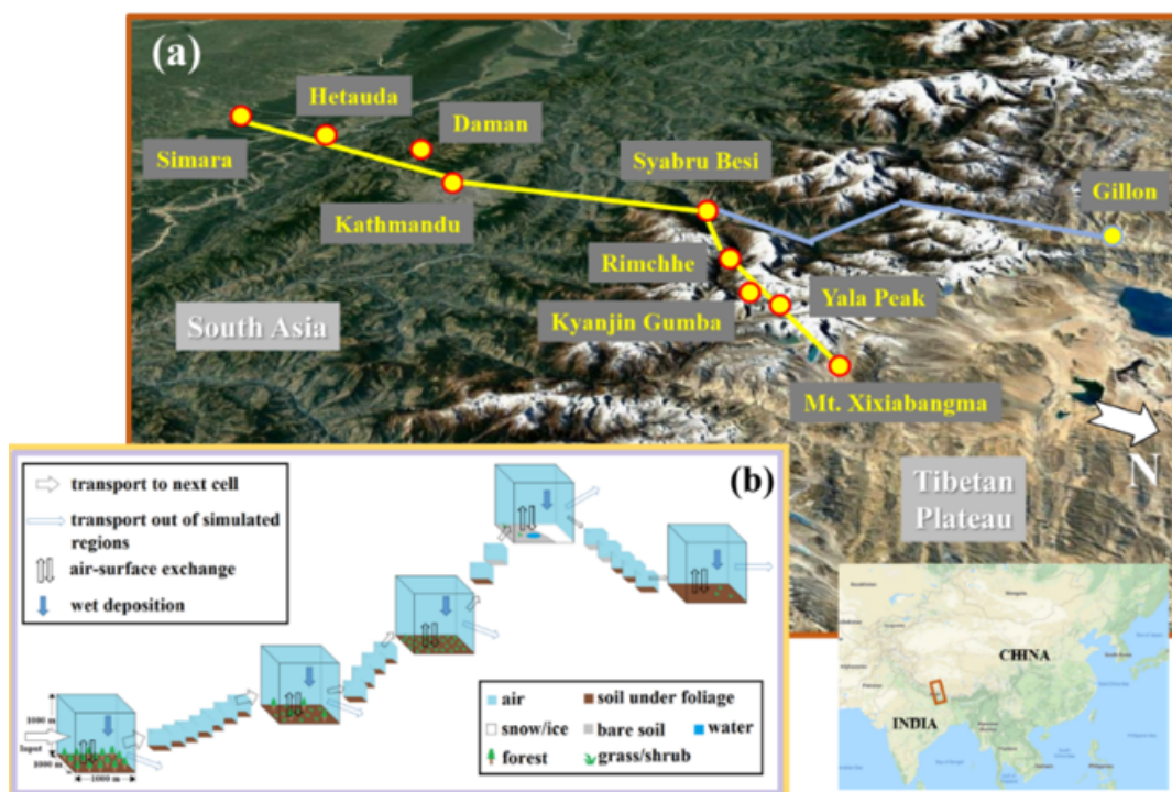
图1. (a)观测和模拟断面;(2)多介质逸度模型概念图
