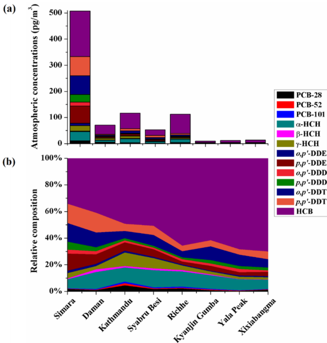
图2. 大气POPs沿山坡传输时的(a)浓度衰减与(b)物质分馏
