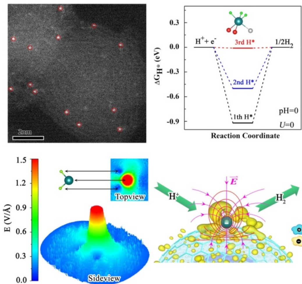
高曲率碳纳米洋葱负载Pt单原子催化剂设计及其析氢(HER)机理
