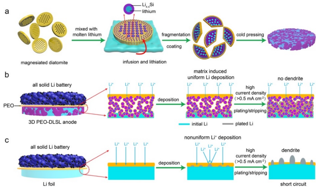
图1：(a)硅藻土模板衍生的多级结构固态锂金属复合负极的制备过程示意图。(b)多级结构固态锂金属复合负极的锂沉积/脱出示意图。(c)平板锂箔负极的锂沉积/脱出示意图。
