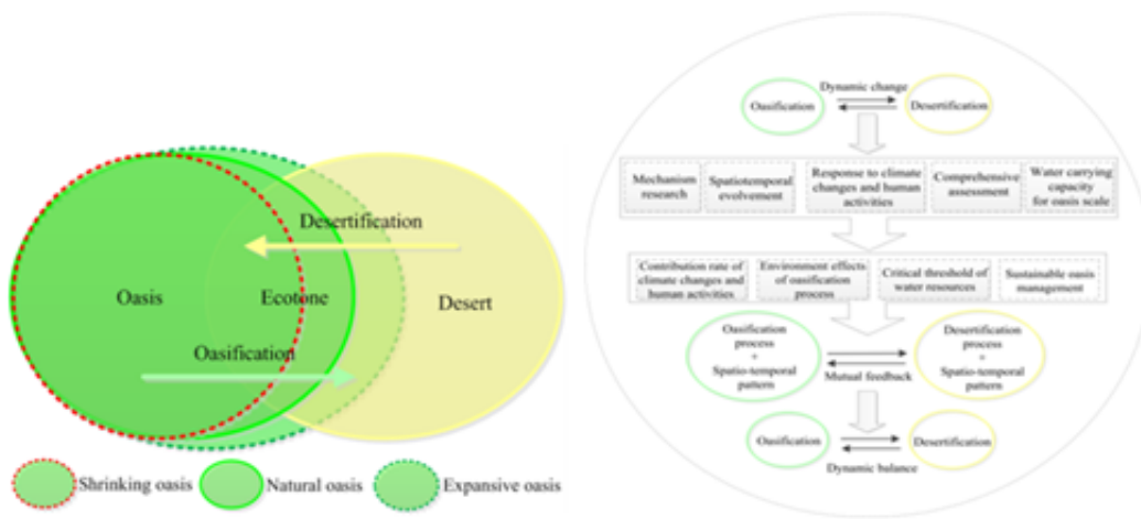
绿洲化与荒漠化博弈过程(左)和绿洲化研究主要框架(右图)
