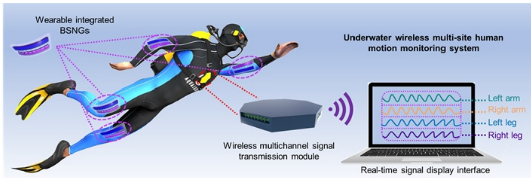
图2 基于BSNG的水下无线运动监测系统
