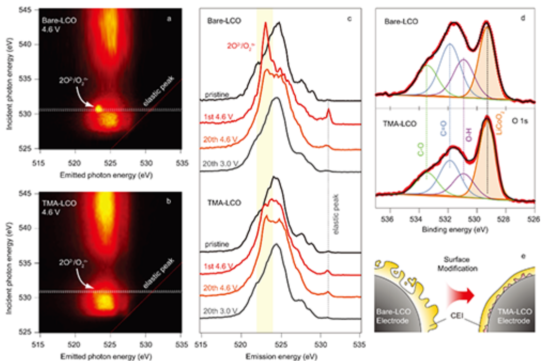
图3. 共振非弹性X射线散射(RIXS)结果表明Ti、Mg、Al掺杂LiCoO 2 材料充电至高电压状态时氧离子的氧化活性被抑制，使得材料具有更稳定的表面
