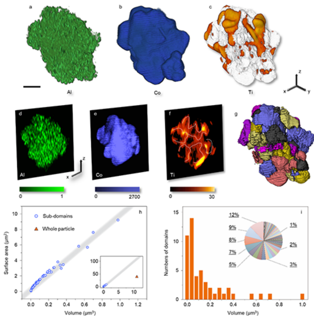
图2. 同步辐射X射线三维成像技术揭示Ti、Al和Co元素在 \text{LiCoO}_2 颗粒中的空间分布
