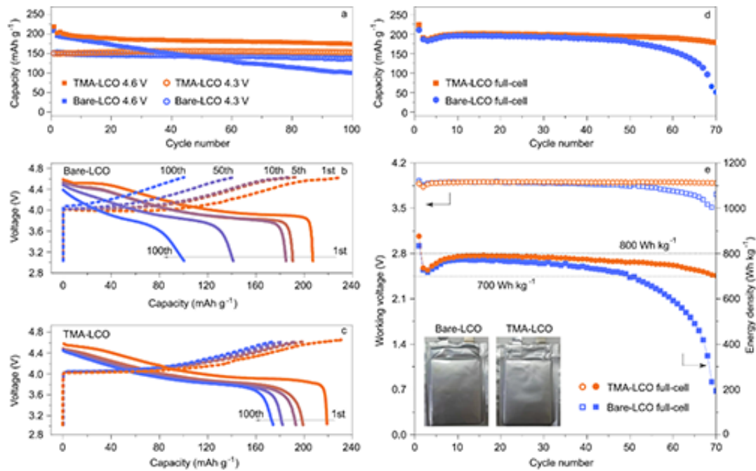
图1. Ti、Mg、Al共掺杂LiCoO 2 (TMA-LCO)与未掺杂LiCoO 2 (Bare-LCO)的半电池和全电池性能对比
