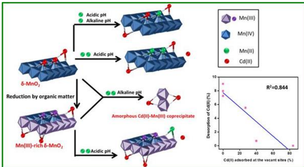
图2 Mn(II)对氧化锰固定Cd(II)的影响机制
