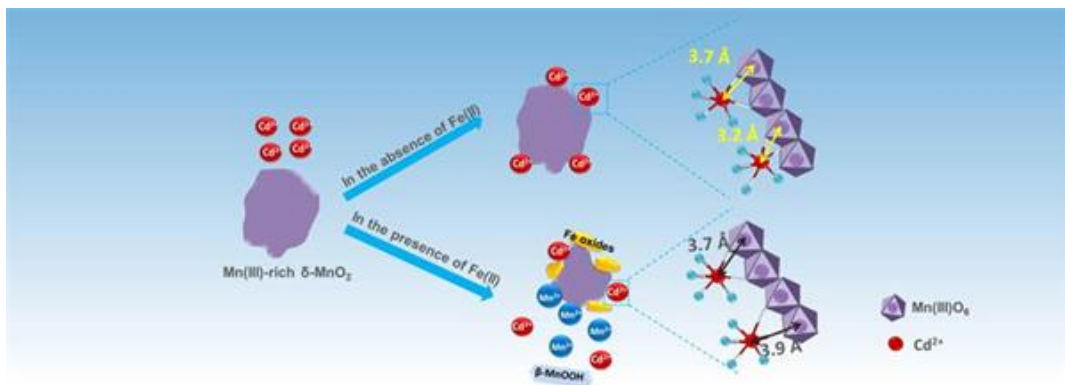
图3 Fe(II)对氧化锰固定Cd(II)的影响机制
