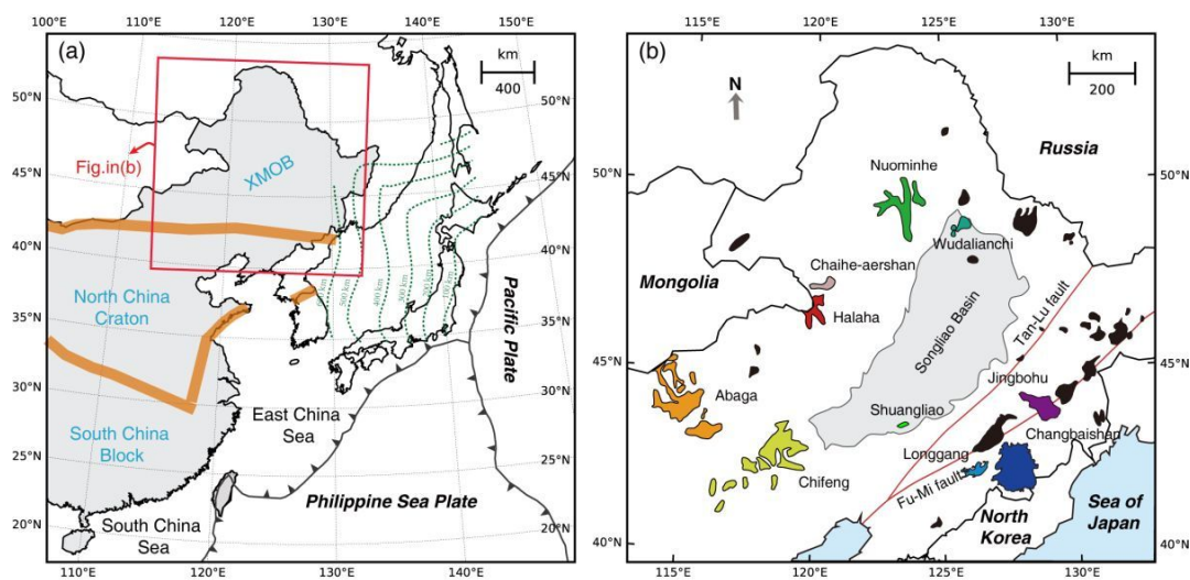
图1(a)东亚板块构造简图。绿色虚线代表太平洋俯冲板片深度等值线(Tang等., 2014)。(b)中国东北地区新生代火山岩分布图(修改自Liu等., 2001)。红色线代表主要断裂。
