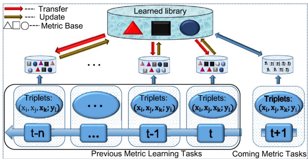
终身度量学习模型
