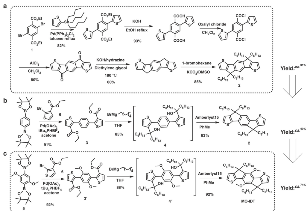
图1 IDIC受体中心稠环核的合成路线简化和优化
