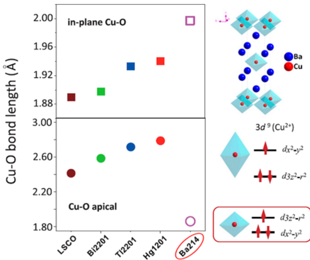
图1. 具有单层铜氧面结构的铜基超导材料的面内氧和顶角氧的铜氧键长、铜氧配位构型、铜的 3d_{x^2-y^2} 和 3d_{3z^2-r^2} 轨道相对顺序。其中La系、Bi系、Tl(Hg)系的顶角氧距离大于面内铜氧键长，呈现拉伸型铜氧六配位构型，导致 3d_{x^2-y^2} 轨道居于 3d_{3z^2-r^2} 轨道之上。Ba214的面内铜氧键长大于顶角氧距离，形成目前唯一的压缩型铜氧配位构型，导致 3d_{3z^2-r^2} 轨道居于 3d_{x^2-y^2} 轨道之上。
