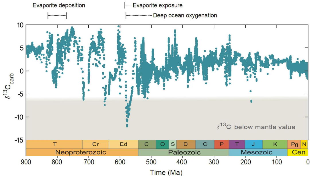
距今9亿年来海水碳同位素( ^{13}\text{C} )记录
