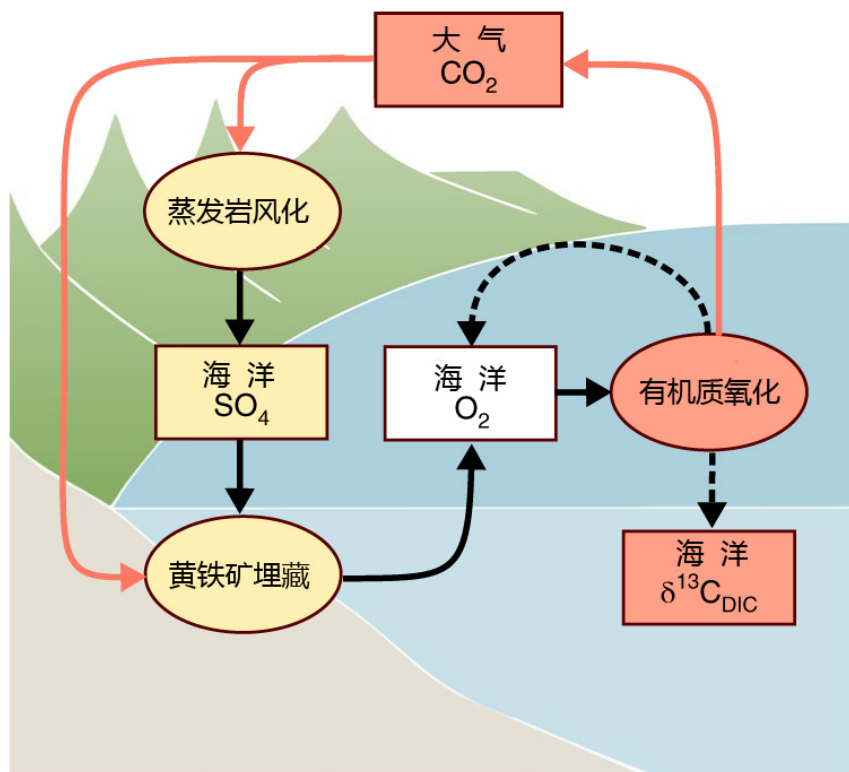
蒸发岩风化与海洋有机碳库氧化的正反馈模型图
