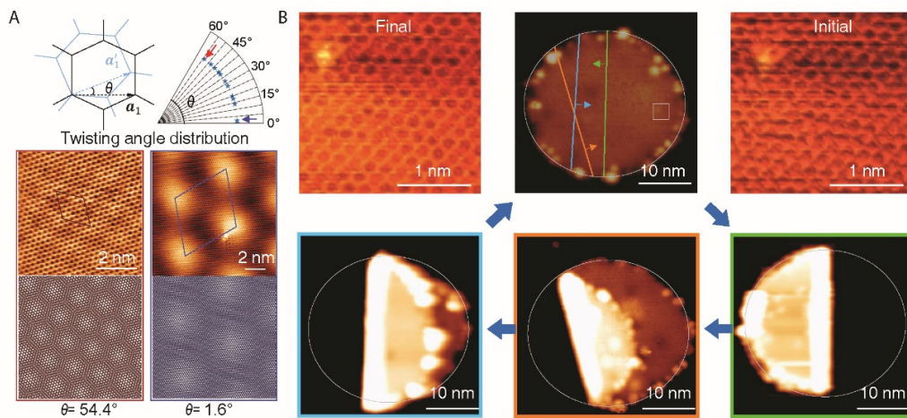
图2 折叠方向精确控制以及角度连续可调的旋转堆垛双层石墨烯的构筑。
