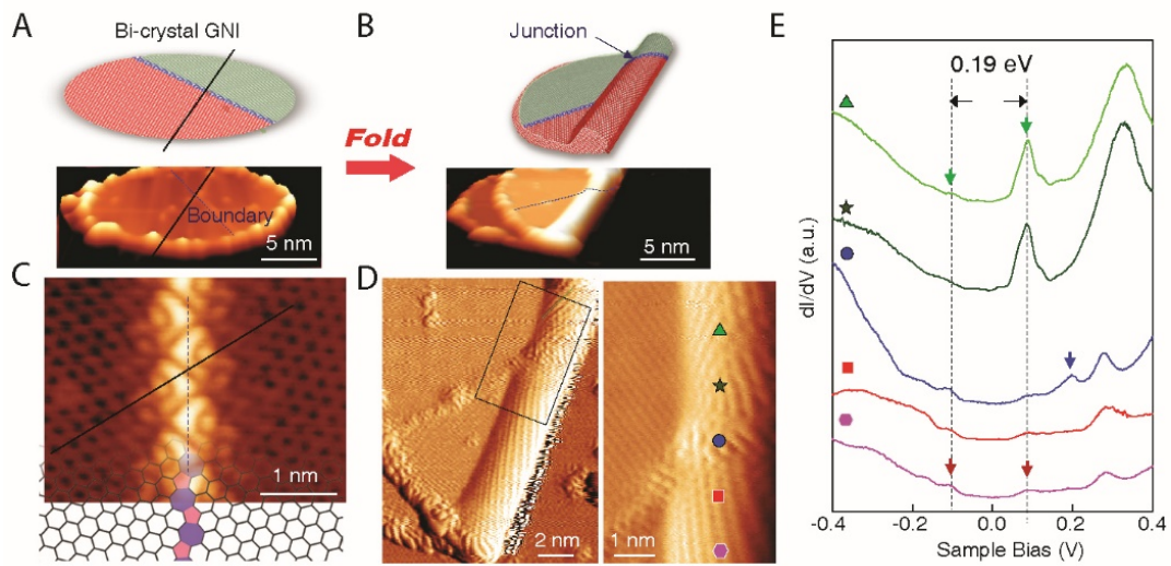
图4 折叠双晶石墨烯纳米片精确构筑异质结构。
