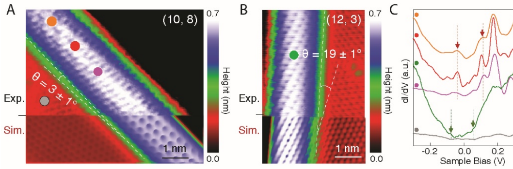
图3 手性结构与电子态精确可调的类一维碳纳米边界结构的构筑。
