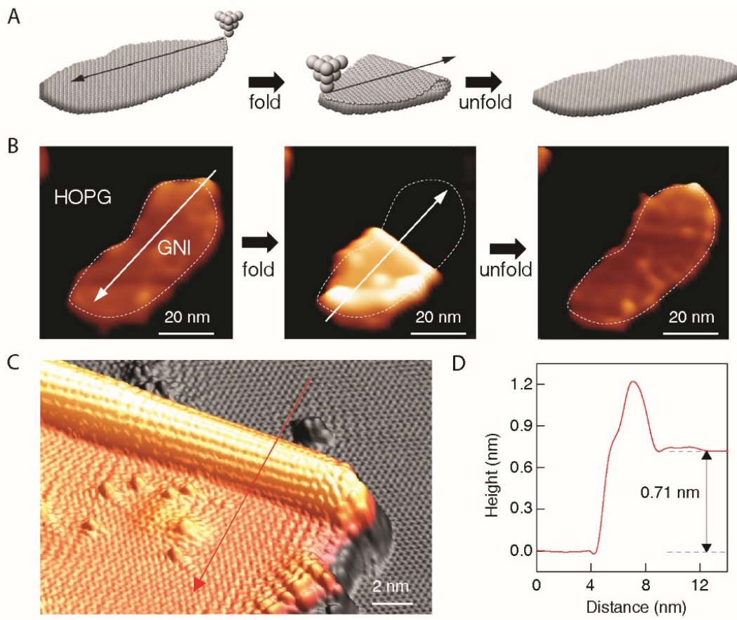
图1 原子级精确石墨烯折纸术构筑三维石墨烯纳米结构。
