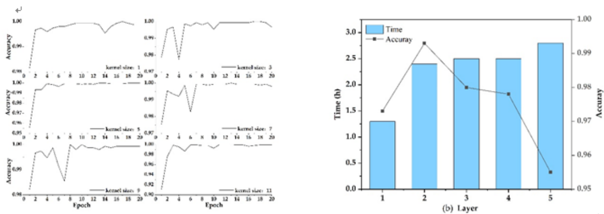
图2 卷积核大小及卷积层数设置对深度学习算法精度及效率的影响
