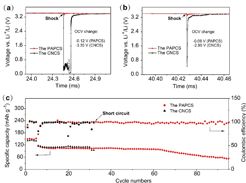
图2.使用商业陶瓷纳米颗粒涂层隔膜和仿珍珠母层隔膜组装的电池的电化学性能对比 该工作提出了构建仿珍珠层增韧隔膜的策略，并从理论模拟和实验测试上证明其提升锂电池抗冲击的能力，这将为今后提升锂电池的安全性开辟新途径。该论文共同第一作者为中国科学技术大学化学与材料科学学院应用化学系硕士生宋永慧与近代力学系博士生吴开金。本研究得到科技部、国家自然科学基金委、中国科学院和国家同步辐射国家实验室的支持。（来源：中国科学技术大学） 相关论文信息： https://doi.org/10.1002/adma.201905711
