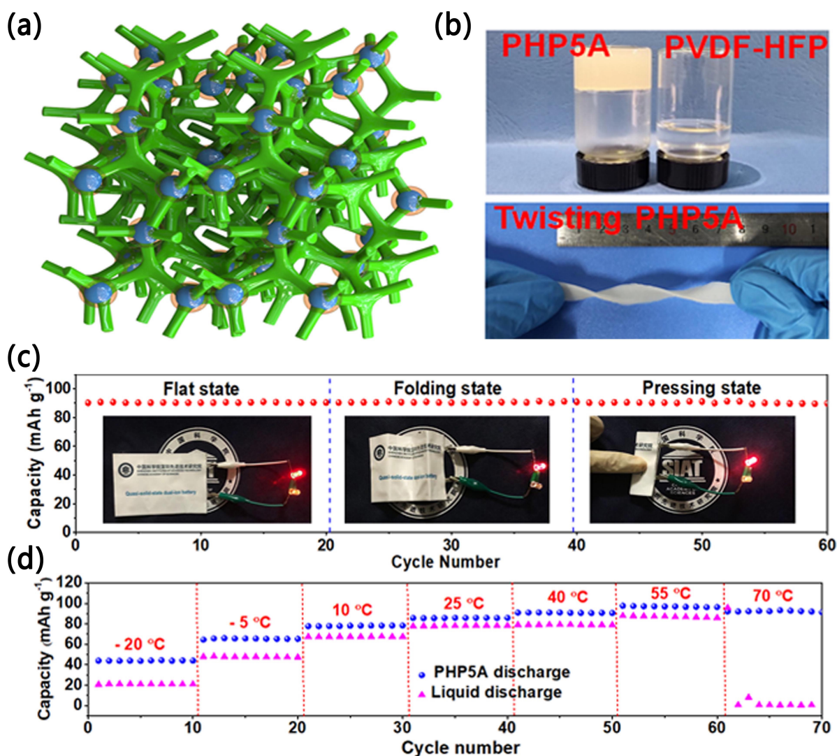
图(a). 由PVDF-HFP和 \text{Al}_2\text{O}_3 纳米粒子之间的路易斯酸碱分子间键合形成的准固态聚合物的3D示意图；(b)准固态电解液和液 态电解液的对照照片（上），准固态电解质扭转实验的光学照片（下）；(c)在平整、折叠和挤 压状态下柔性SDIB的循环曲线；(d)在-20-70 °C，基于准固态电解液和液态电解液循环性能对比 。 研究团队单位：深圳先进技术研究院
