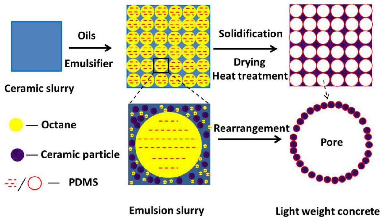
试样制备流程图
