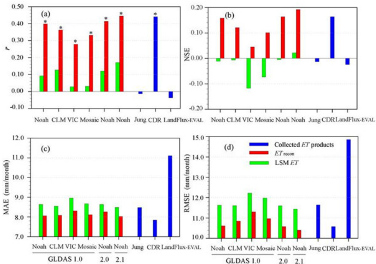
图：黄河流域重建蒸散发的检验，红色bar代表基于GLDAS模式重建蒸散发的统计结果，绿色bar表示基于GLDAS模式原有蒸散发的结果，Jung、CDR及LandFlux-EVAL为收集的蒸散发数据产品，图中的统计指标均利用去除季节循环后的蒸散发序列计算得到，*表示通过95%显著性检验。
