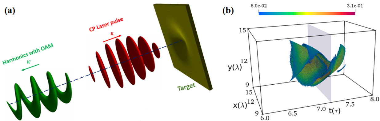
图1 圆偏振光转化为涡旋光的原理图和单个阿秒涡旋脉冲的空间结构示意图
