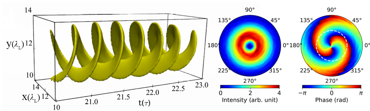
图2 三阶谐波的相位结构以及强度分布
