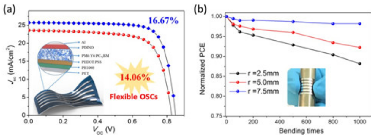
图2 (a) 电池结构示意图和J-V曲线，(b) 不同半径 ( r = 2.5, 5.0 和 7.5 mm) 弯曲测试后的效率变化
