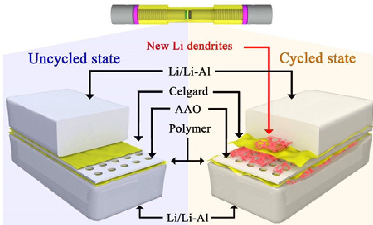
图：无损、原位同步辐射X射线三维成像技术研究锂金属电极工作机制
