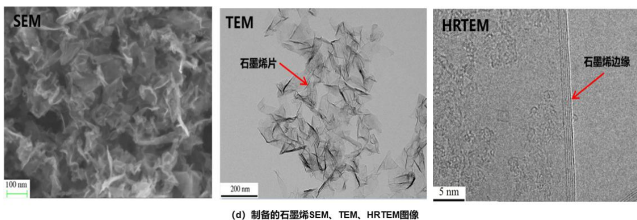
图：不同模式电弧CCD图像与石墨烯样品检测结果
