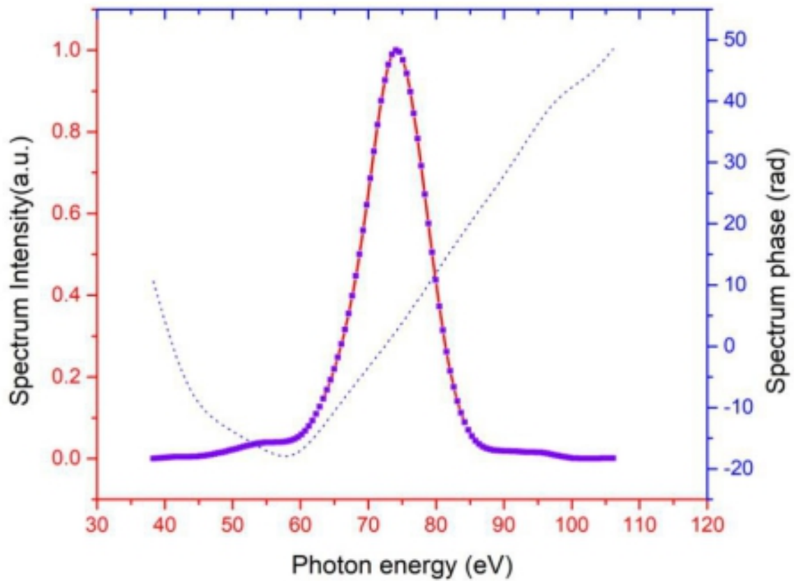
阿秒脉冲光谱及相位分布
