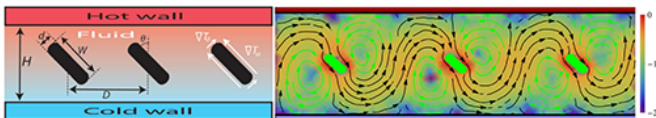
图2：（左图）温度梯度驱动的微流泵示意图。棒状胶体粒子固定于充满液体的微通道内，通道上下边界墙具有不同的温度。胶体粒子受到一个垂直于温度梯度（即平行于通道）的热泳力。（右图）动力学模拟所得到的流场。固定胶体棒所受到热泳力的反作用力驱动周围流体的定向流动，黑箭头表示净流场，绿箭头表示蜗旋流场，颜色代表流速。
