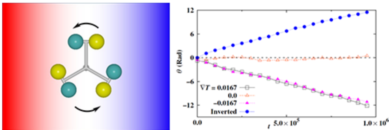
图1：（左图）扩散流驱动的微涡轮机示意图。三对哑铃状粒子所构成的手性胶体结构处于梯度场之中，不同的粒子颜色代表不同材料，外加的梯度场可以是热或者化学梯度。该手性结构受到一个垂直于梯度场的泳力矩。（右图）动力学模拟所得到的涡轮机转角与时间的关系。在泳力矩的作用下，该胶体结构绕其中心、垂直于梯度场单向地转动。转速大小依赖梯度场的幅度，转动方向仅取决于胶体结构的手性而与梯度方向无关。
