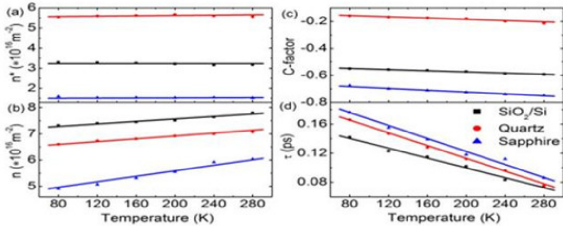
图1. 三种不同衬底上单层MoS 2 的 (a) 有效电子浓度, (b) 电子浓度, (c) 电子局域化因子, (d) 电子弛豫时间随温度的变化关系。实验结果由太赫兹时域光谱测量得到。
