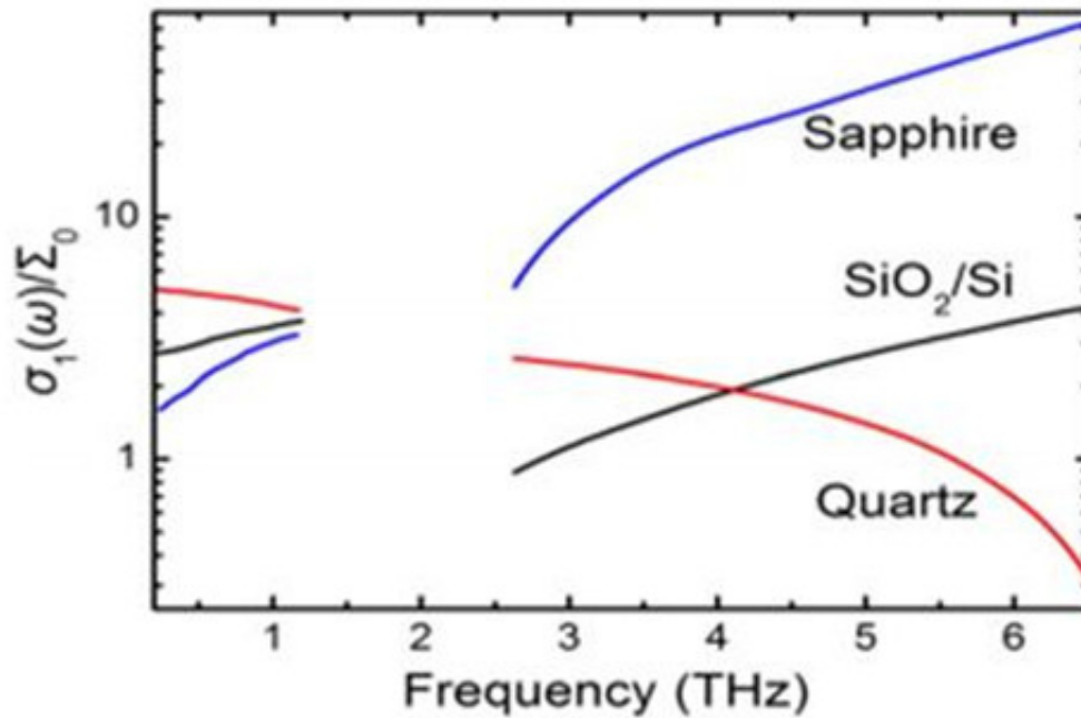
图2. 室温下单层MoS 2 在SiO 2 /Si、蓝宝石、石英衬底上的光电导率实部随频率的变化关系。低频结果由太赫兹时域光谱测量得到, 高频结果由太赫兹傅里叶光谱测量得到。
