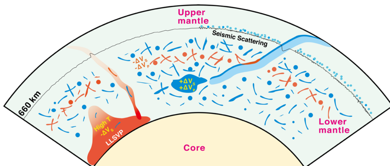
图2 俯冲洋壳与下地幔波速异常体的关系示意图
