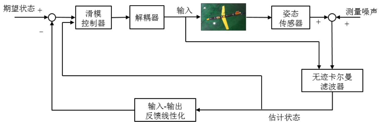
基于无迹卡尔曼滤波器的滑模控制系统
