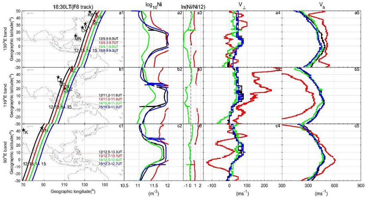
图3DMSP F8卫星经过130 ° E、110 ° E和90 ° E观测到的840 km电子密度Ni与垂直轨道速度V。不同颜色代表不同日的观测结果：红色为13日磁暴主相，绿色为14日恢复相，黑色为12日暴前，蓝色为暴后15日
