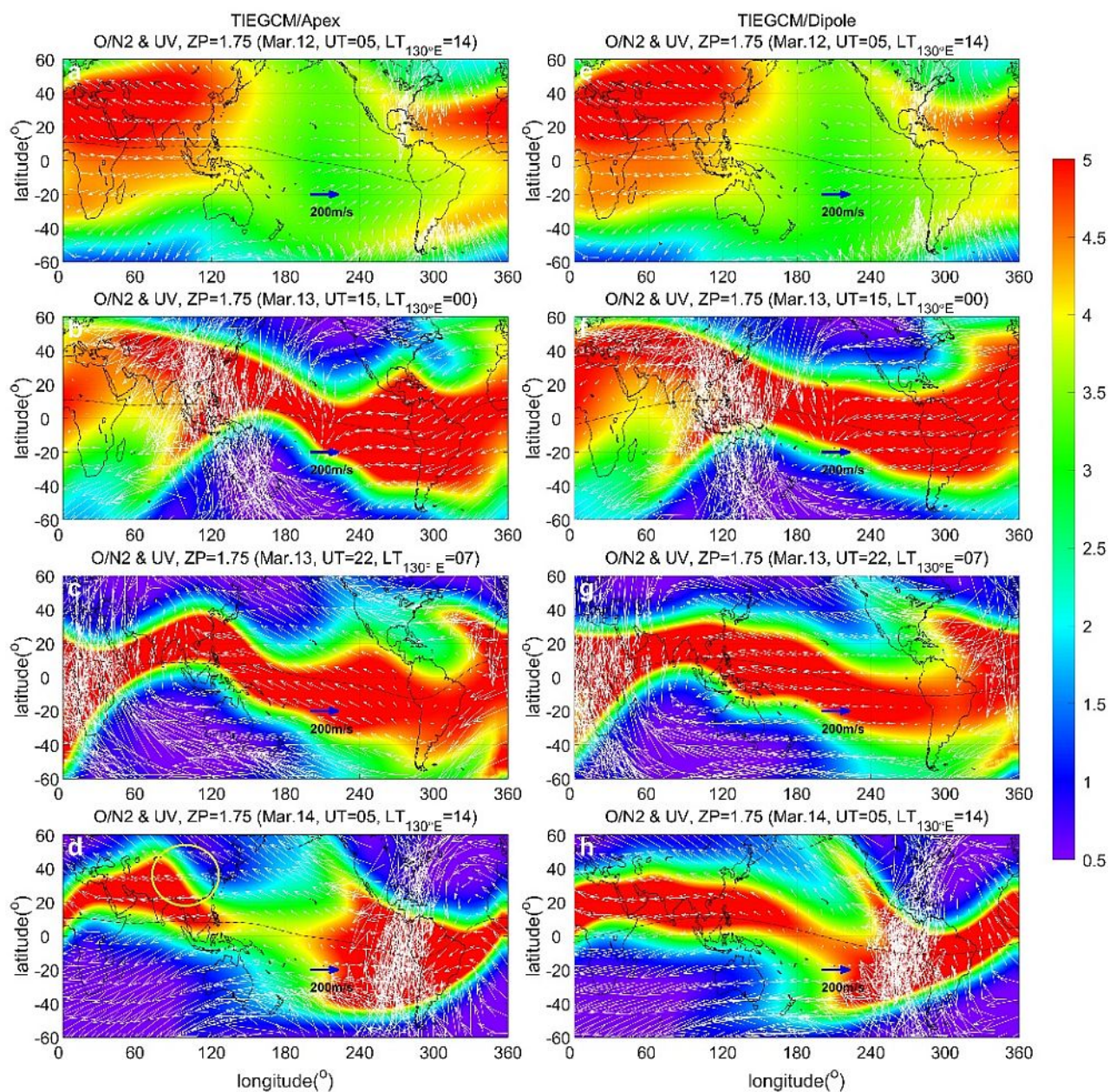
图4 真实地磁场（左）和偏心偶极场（右）下的TIEGCM模拟结果O/N2UV
