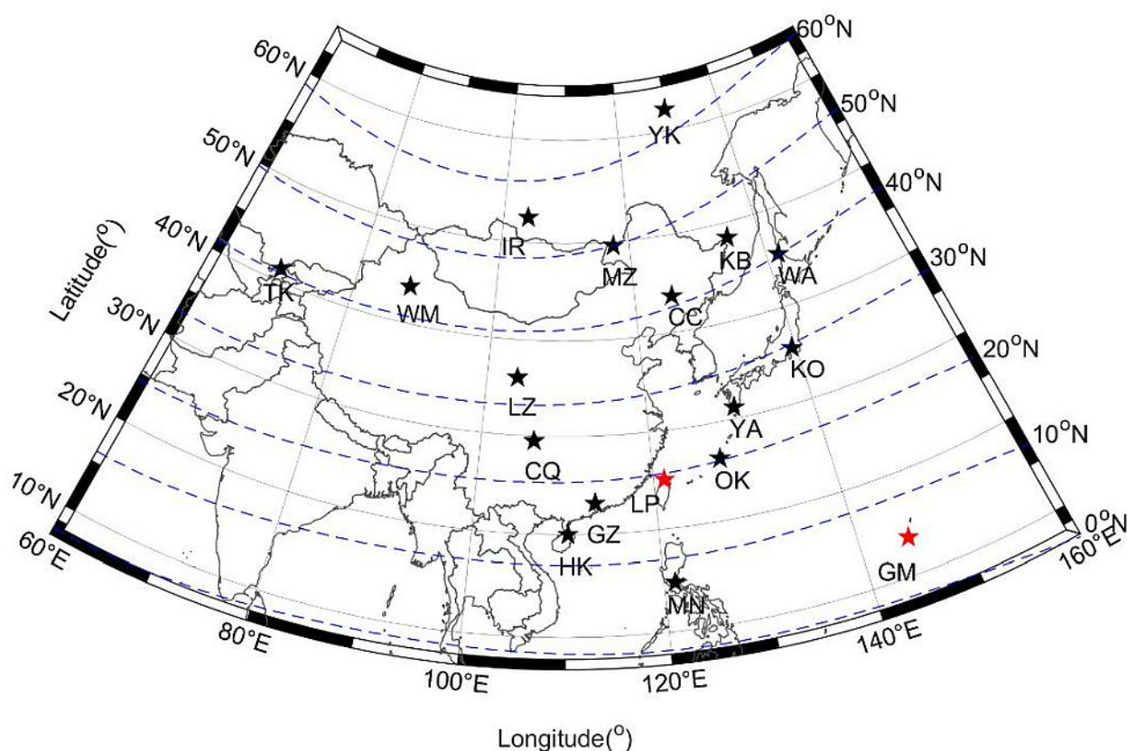
图1 中国及其周边地区的测高仪观测台站的地理分布
