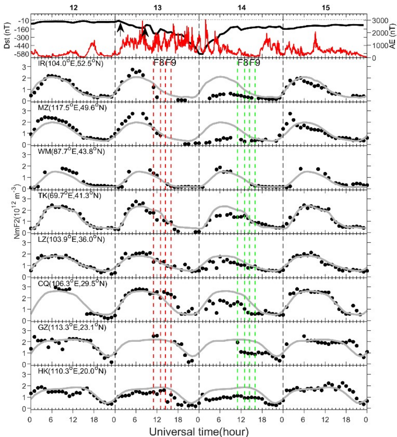
图2 东部地区测高仪观测NmF2 (上) 和中西部地区测高仪观测的NmF2 (下)。上：东部扇区的电离层台站从中纬度到磁赤道地区 (YK, KB, WA, CC, KO, YA, OK和MN) 在磁暴主相和恢复相期间 (13日12 UT ~ 14日18 UT) 其F2层峰值密度均出现长时间大幅度下降, 持续时间超过24个小时。下：西部扇区的电离层台站只在中纬度地区出现大幅下降, 如IR, MZ等台站, 而靠近中国中西部地区的WM, TK, LZ其下降幅度与东部同磁纬的台站相比并不显著, 低纬台站CQ, GZ和HK站其下降幅度也均小于东部扇区的同纬度台站。
