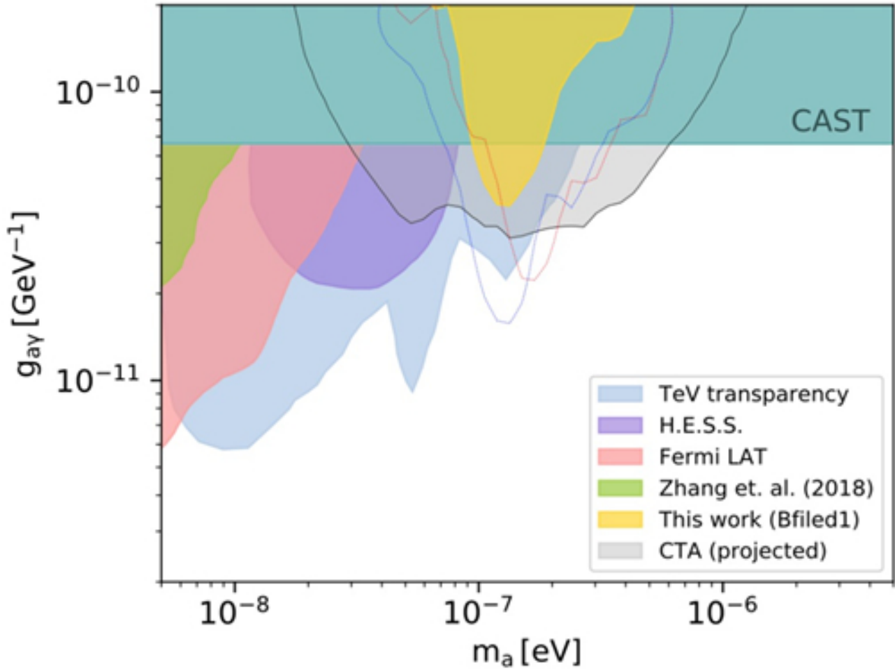
图：目前对类轴子质量 ( m_a ) 和耦合常数 ( g_a ) 参数空间限制的比较。其中黄色区域为本项研究得到的排除区域 (95%置信度)。红、蓝两条虚线分别代表选取另外两个不同的银河系磁场模型时对参数空间的限制。蓝色区域为解释TeV transparency 理论预言的类轴子参数空间。
