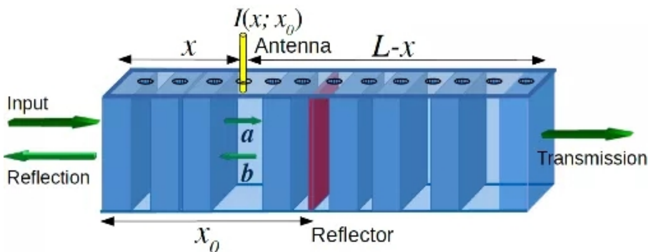
微波实验示意图
