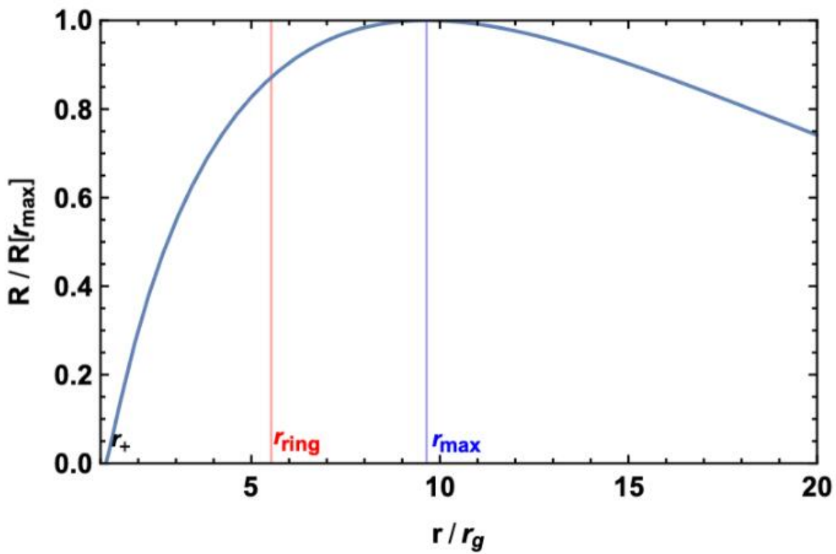
图1：轴子云波函数在径向方向上的大小
