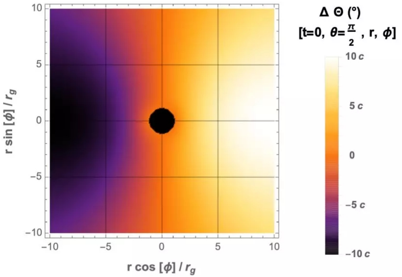
图2：同一时刻轴子引起的偏转角偏移在黑洞赤道平面上的投影
