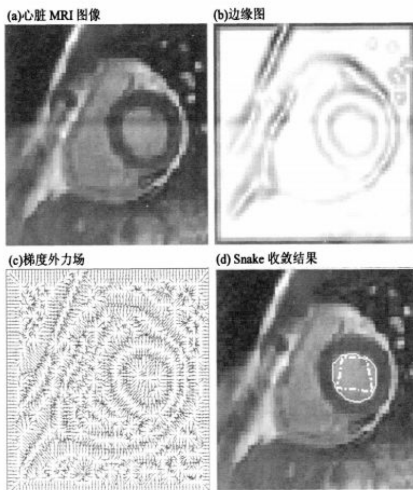
图 2-1 传统 Snake 对心脏 MRI 图像分割结果
