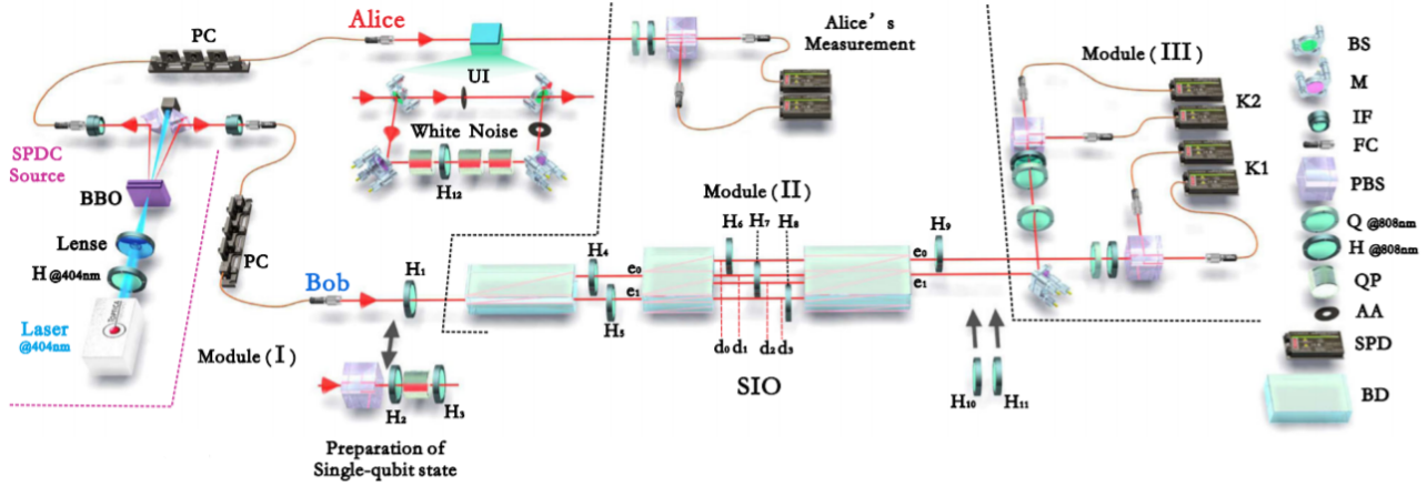
图1：实现量子态非相干转化的实验装置图
