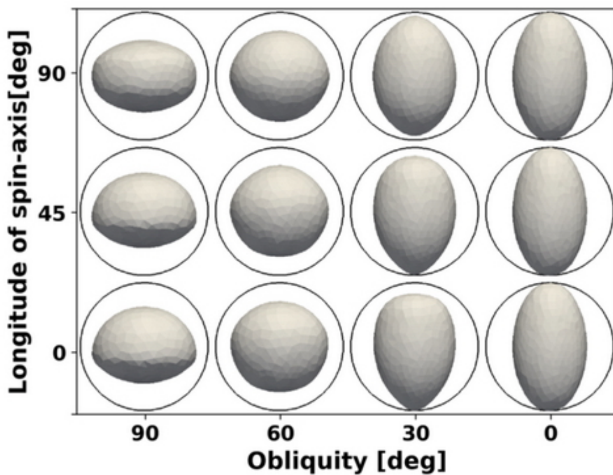
图2在相同的动力学轨道上，不同自转轴指向的球形彗核在CO挥发作用下的形状演化结果。
