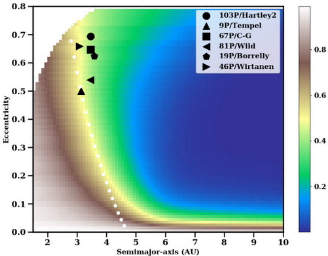
图3 不同轨道构型下，单位面积水分子在远日点半轨道和近日点半轨道挥发总量的比值。不同的黑色形状标记目前人类探测器造访过的木星族彗星，白色曲线对应远日点在气体生产率曲线拐点位置的轨道。当远日点位于气体生产率曲线拐点位置以外时，彗核形状在物质挥发作用下产生南北差异的现象开始显现；当该比值大于0.5，该现象相对较为显著。
