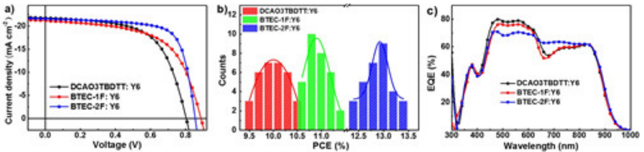
图2 a) 器件J-V曲线；b) 全小分子电池效率统计分布图；c) 器件的EQE曲线
