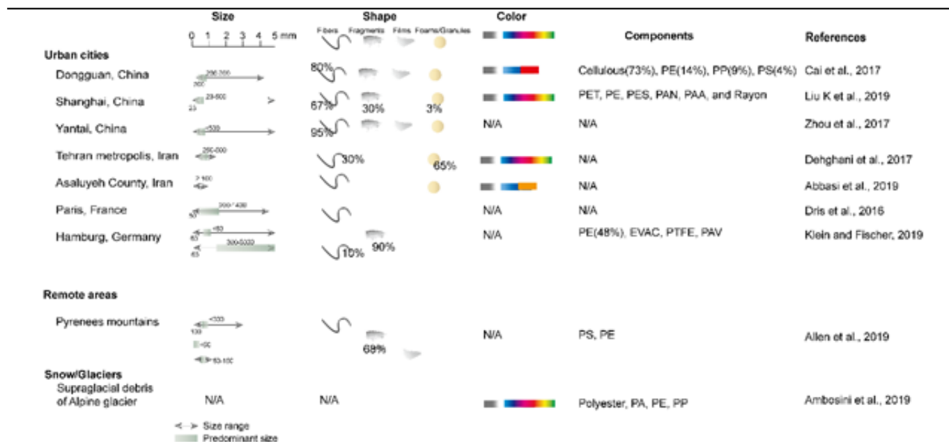
图2 大气微塑料尺寸、形状、颜色和组成等特征总结
