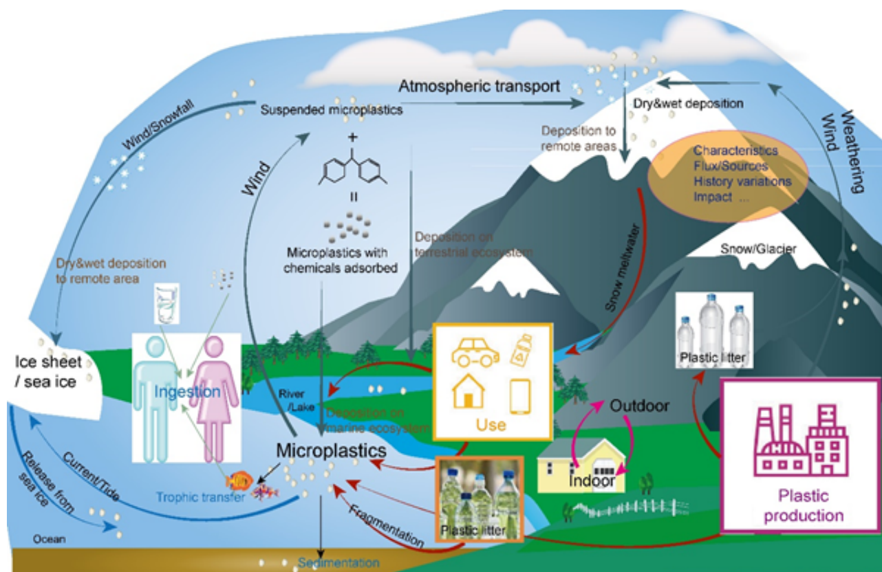
图3 环境中大气微塑料概念图
