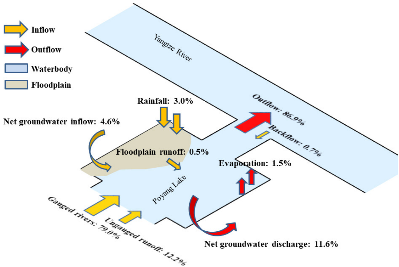
图1 鄱阳湖洪泛系统水量平衡示意图
