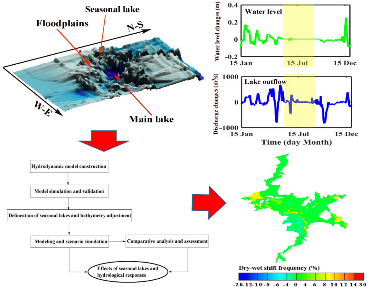
图2 鄱阳湖水文连通性的水动力影响
