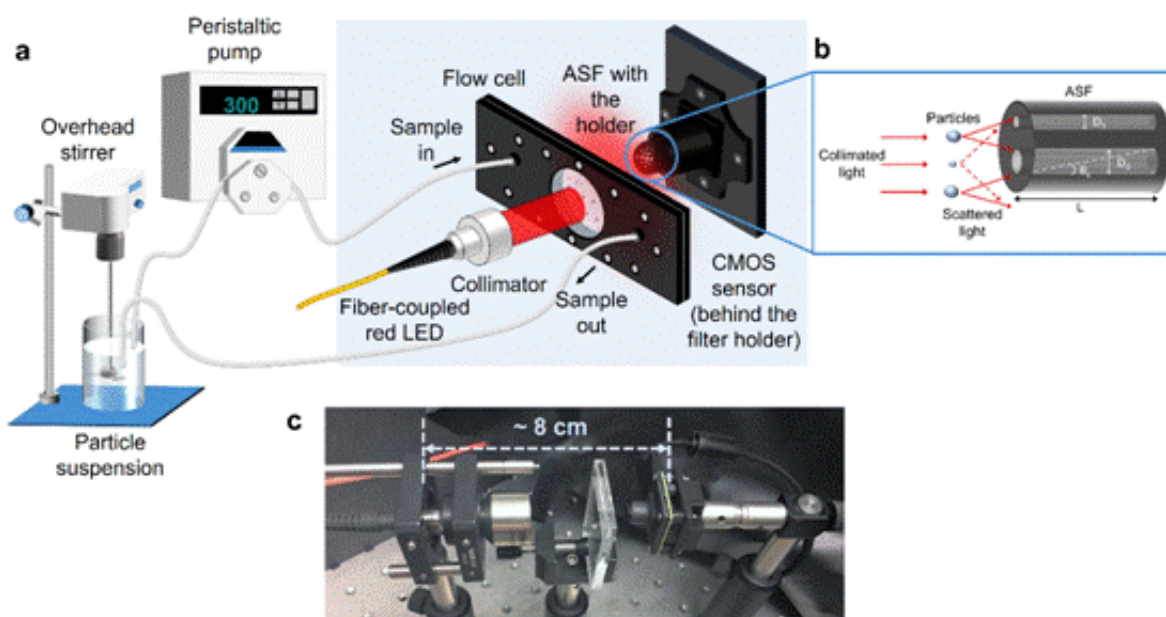
图1：基于机器学习的粒径分析仪的工作原理 (a)测量颗粒悬浮物的实验装置示意图，显示了由耦合LED的光纤、CMOS图像传感器摄像机和聚合物角空间滤波器(ASF)组成的光学硬件。(b) ASF的工作原理: 将粒子样品中的散射光收集到特定的累积截止角，截止角由孔的几何尺寸确定。为了简单起见，只表示了两个孔，但是在最初的实验中使用了23个不同直径(即截止角)的孔。(c) ICFO中光学硬件实验室原型。
