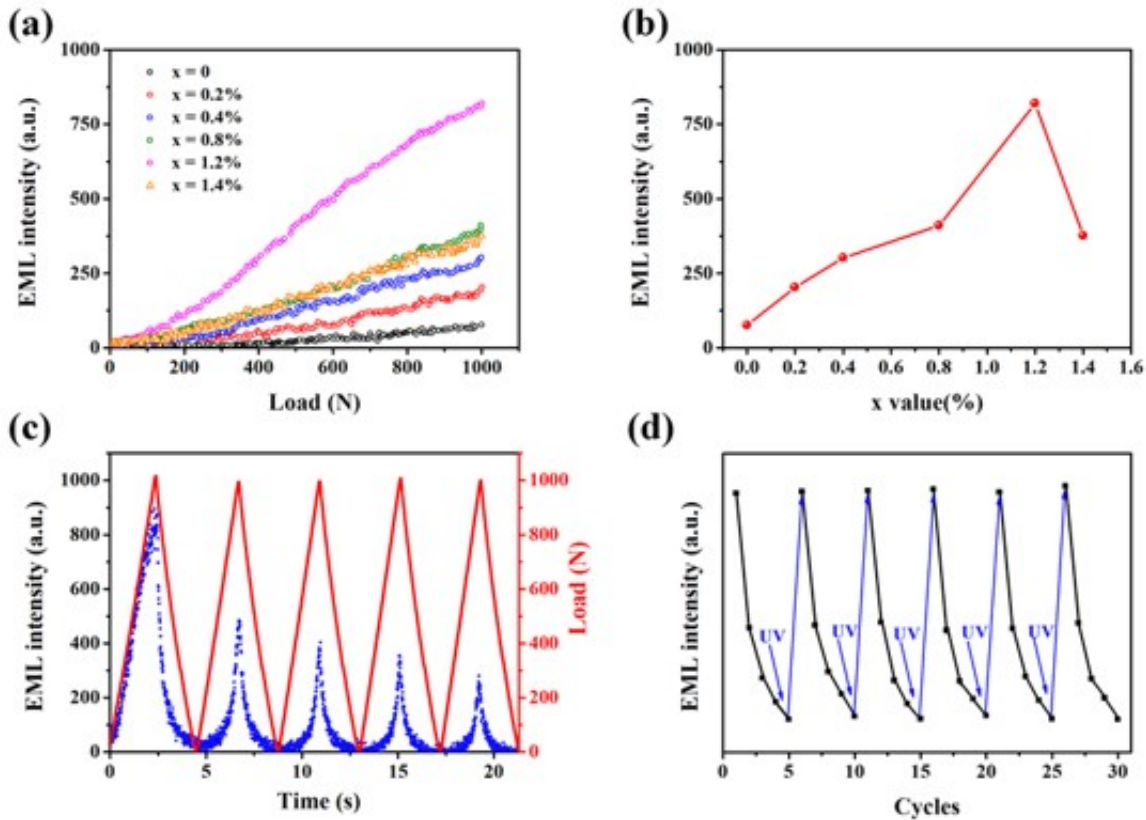
(a)CaZnOS : Mn 2+ , Nd 3+ 在不同Nd 3+ 掺杂浓度情况下的弹性应力发光强度变化；(b)在压缩负荷为1000 N时所有样品弹性应力发光强度与对应x值的关系图；(c)ZnO : Mn 2+ , 1.2%Nd 3+ 在5次重复压力下的弹性应力发光强度变化情况；(d)在紫外线照射后弹性应力发光强度恢复行为。
