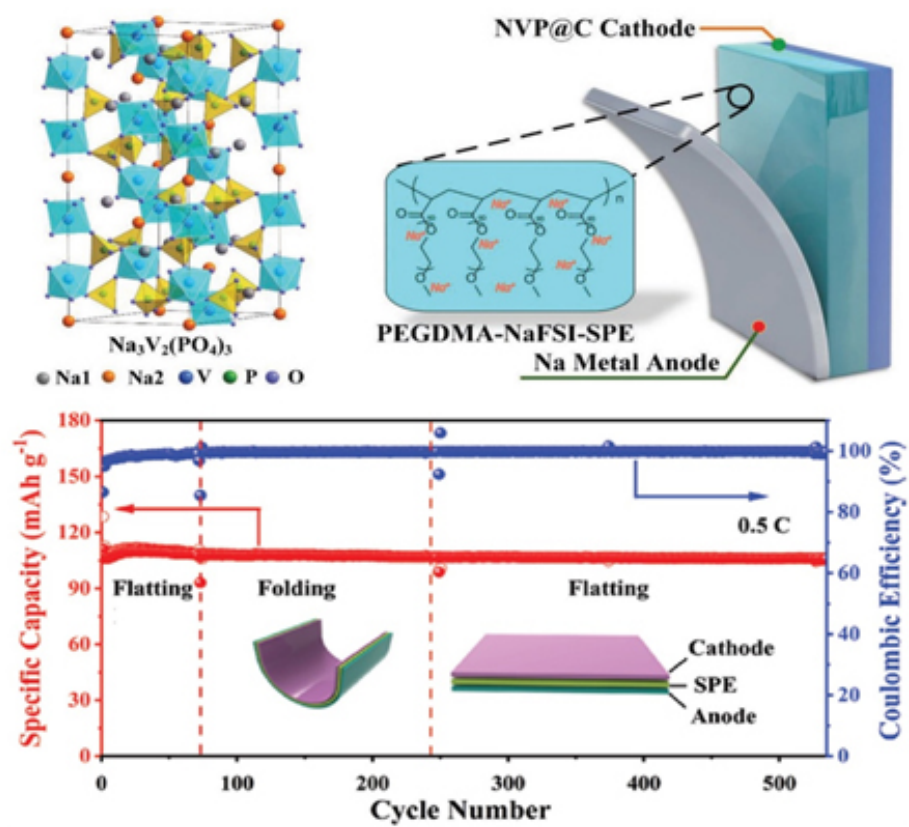
柔性全固态钠电池示意图和循环稳定性
