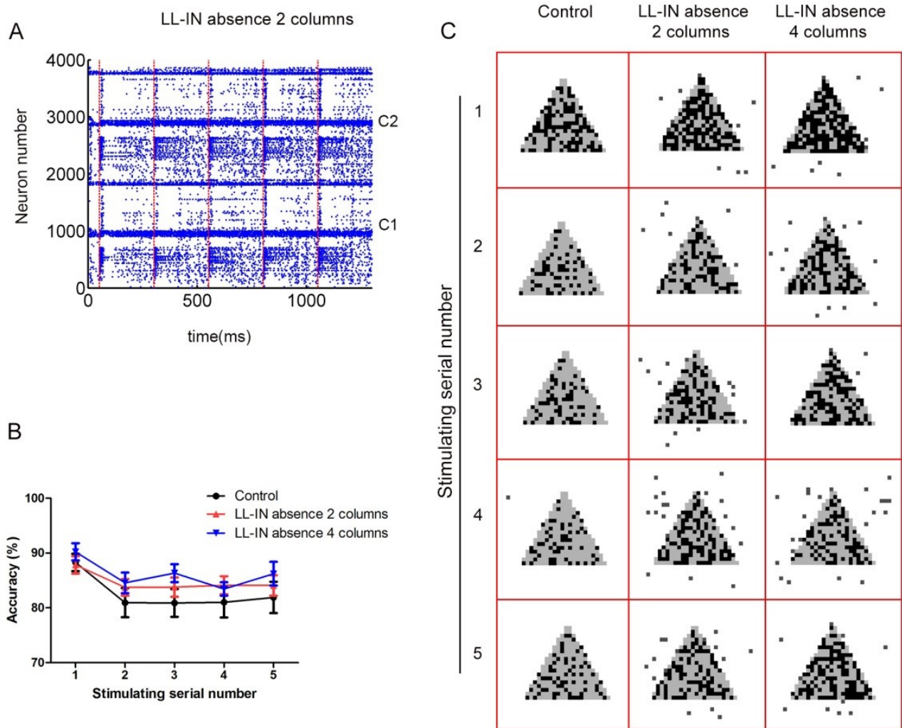
图4 多功能柱网络局部抑制神经元缺失下网络的输出（A，C）与准确率统计分析（B）
