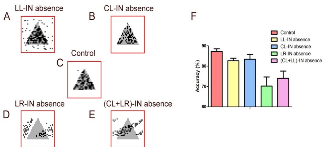
图2 不同类型中间神经元缺失的输出结果 (A-E) 和准确率统计分析 (F)
