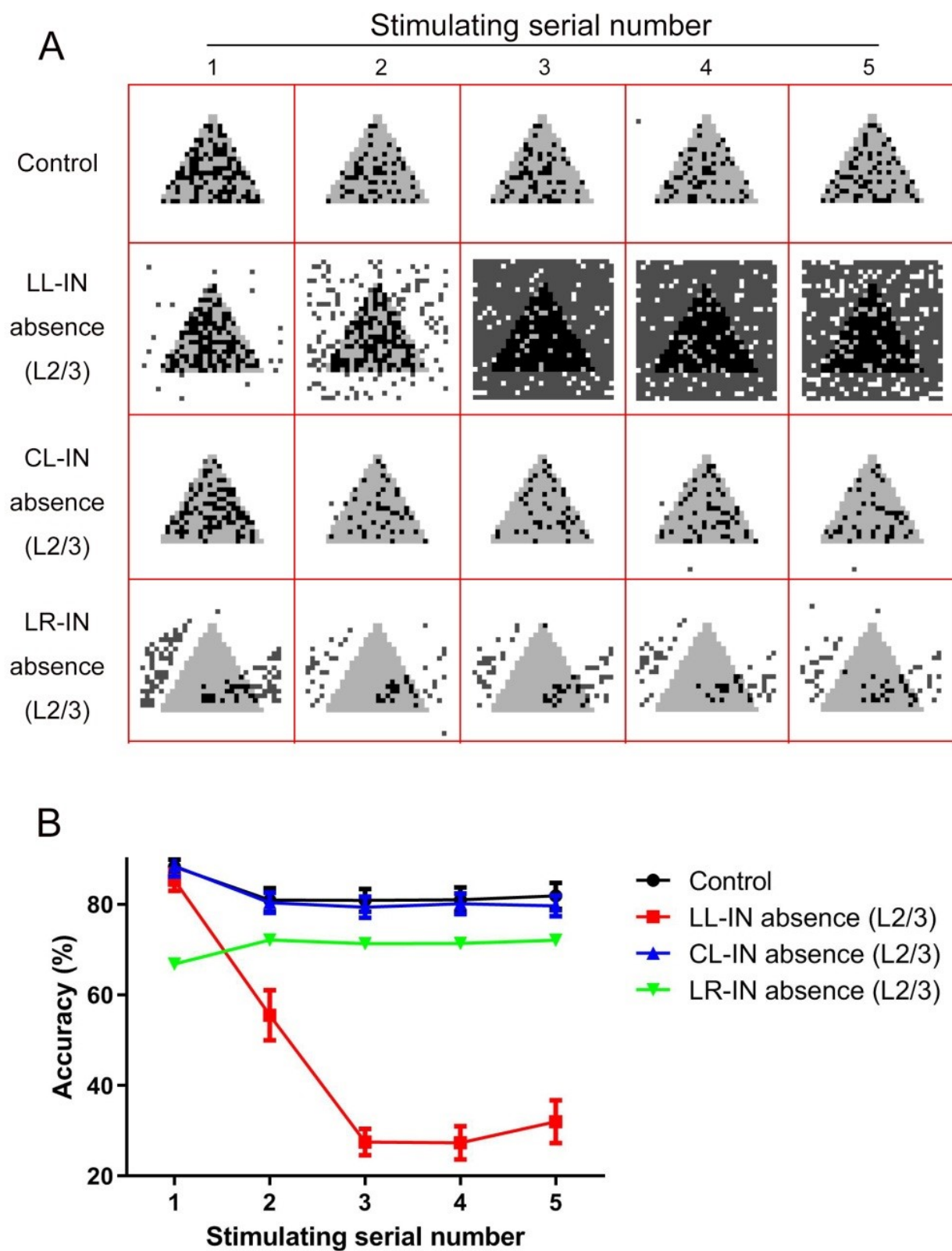
图3 多次刺激下不同类型中间神经元缺失情况下网络的输出 (A) 与准确率统计分析 (B)
