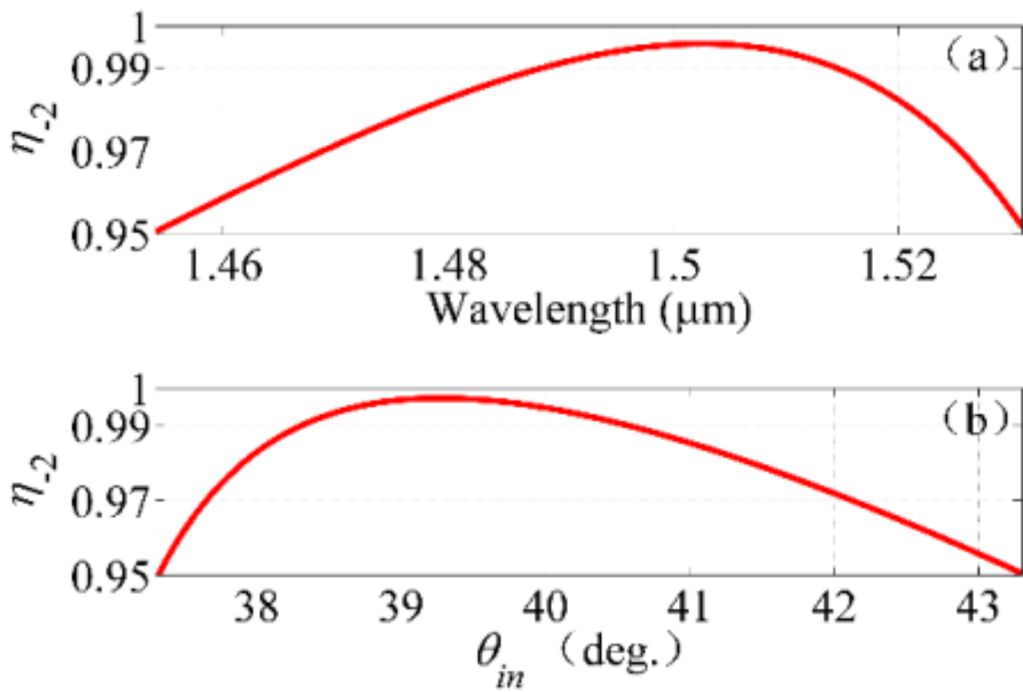
图2 TE偏振入射下行射效率分别随波长(a)、入射角度(b)变化示意图
