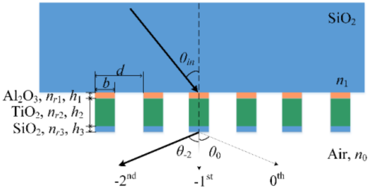
图1 三层全介质矩形光栅示意图
