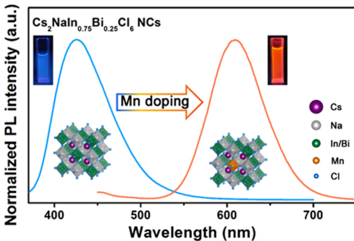
锰掺杂对钠基非铅双钙钛矿纳米晶发射光谱的影响
