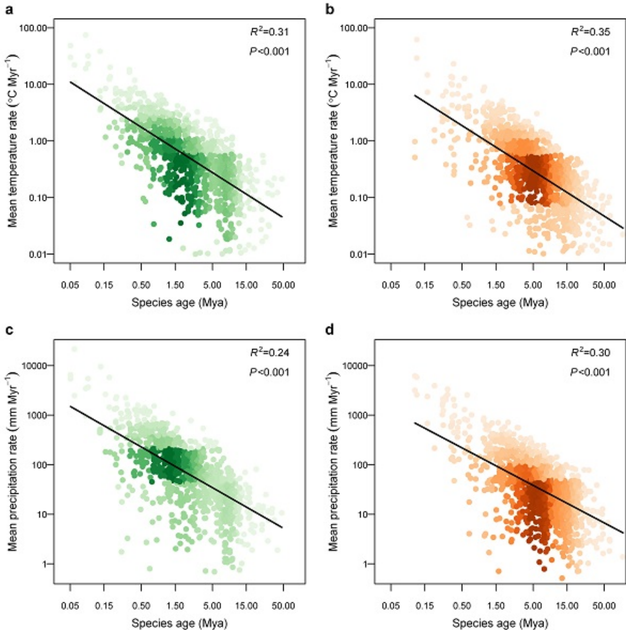
图：全球尺度植物和动物类群气候生态位演化模式的相似性。此为十个假设中的一例，即植物(绿色, n=952)和动物(橙色, n=1135)类群中，物种形成时间越短、气候生态位演化速率越高。(a-b)温度生态位演化速率;(c-d)降水生态位演化速率，颜色深浅代表数据密度，R 2 和P值基于PGLS系统发育模型。
