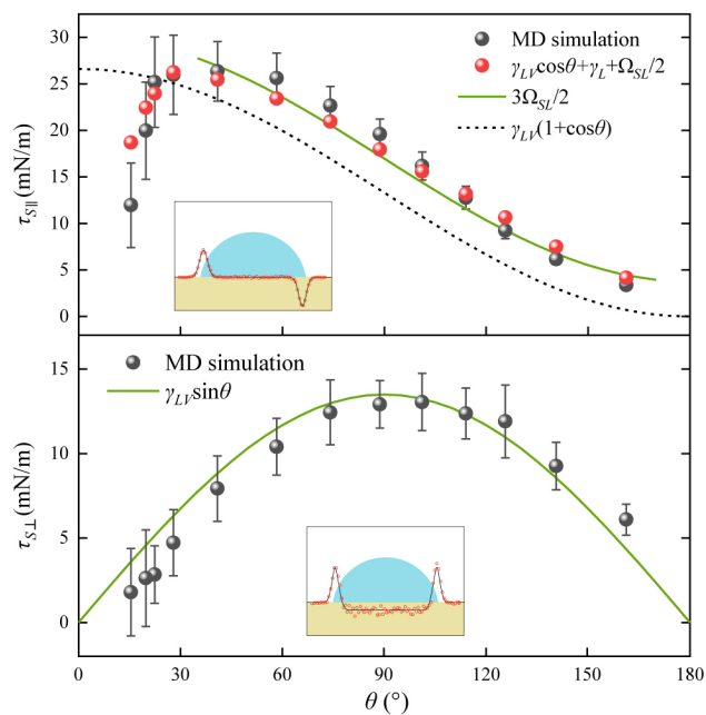
液滴三相接触线处毛细力平衡的理论模型与验证
