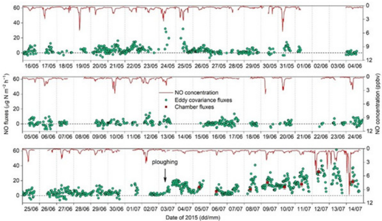
半小时平均的一氧化氮浓度和湍流通量
