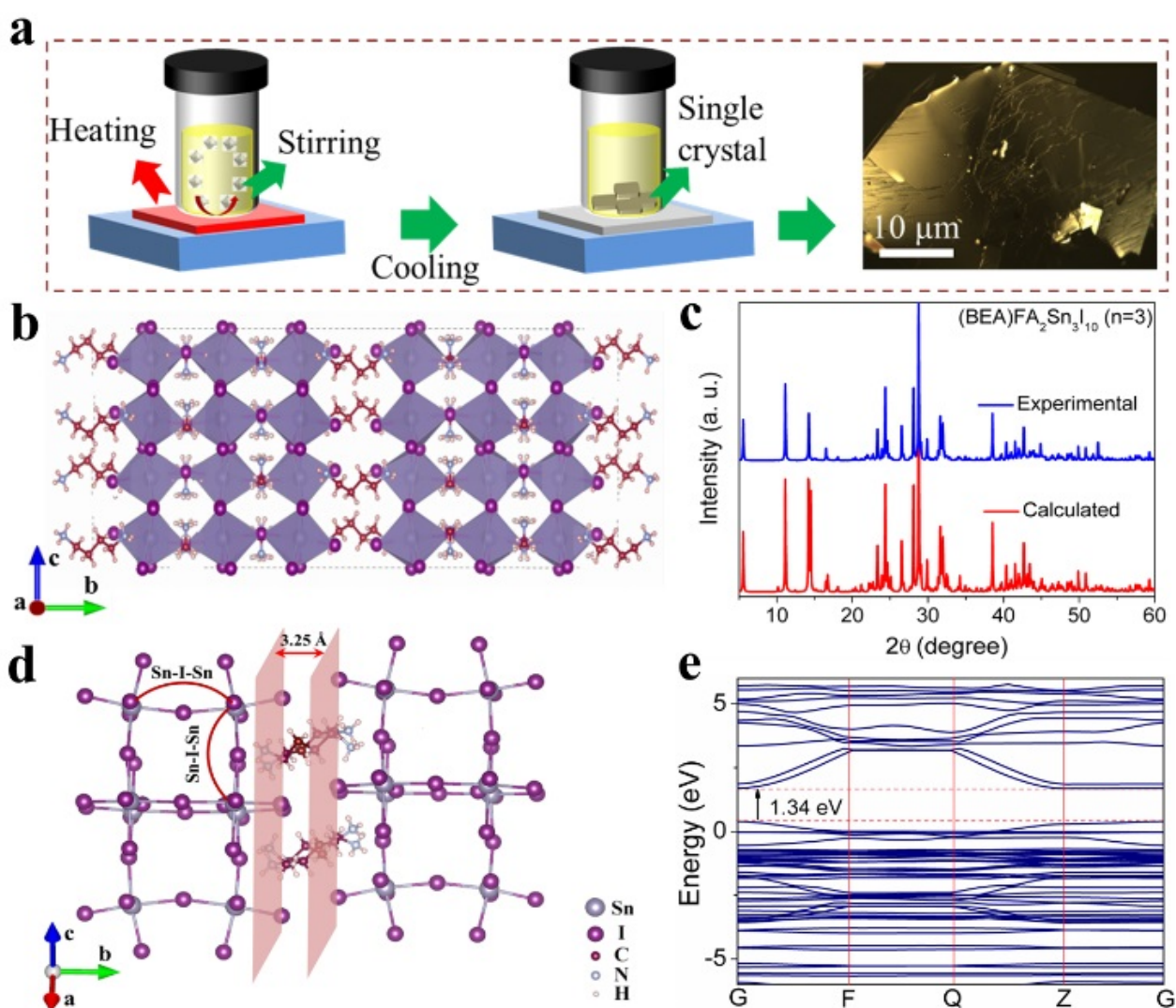
单晶(BEA)FA 2 Sn 3 I 10 的合成，晶体结构及第一性原理计算
