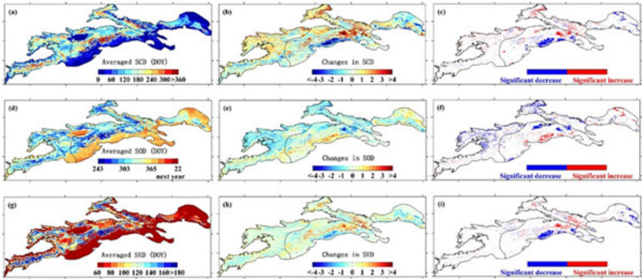
天山地区2002/03-2017/18期间积雪天数(a,b)积雪开始时间(d,e)和积雪结束时间(g,h)的多年平均和变化趋势,(c,f,i)分别为各自的置信水平
