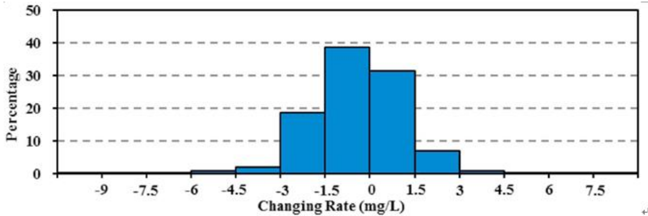
图1 研究区水体TSM浓度变化率直方图
