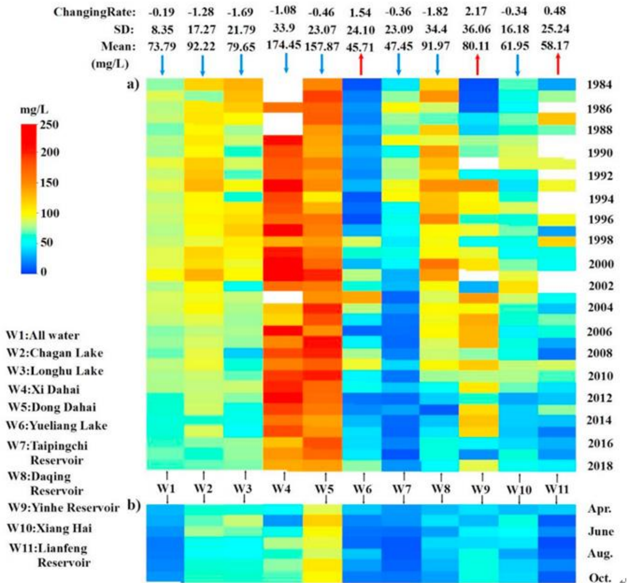
图2. (a) 研究区1984年至2018年水体TSM浓度年度序列，(b) 月平均TSM浓度序列（4月至10月）
