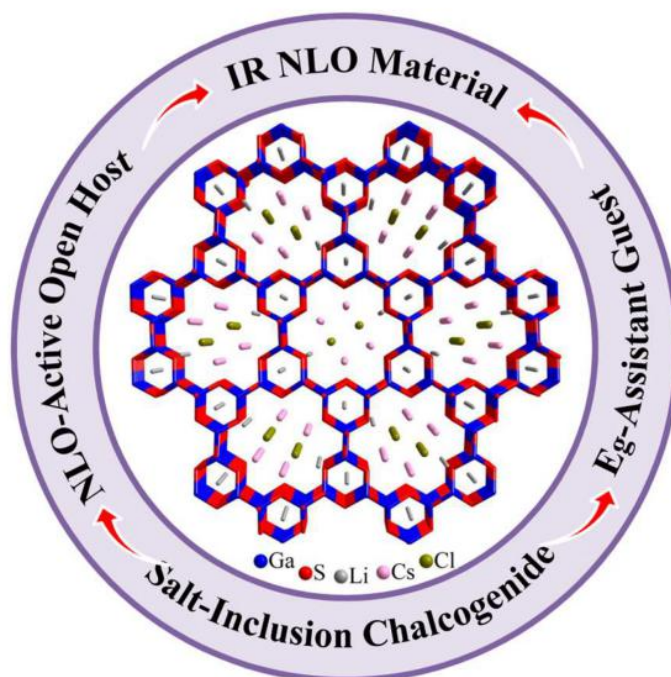
图：双“功能基元”协同作用获得优秀的红外NLO晶体材料
